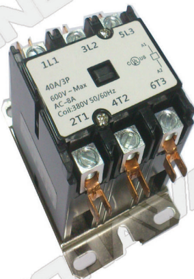
แมกเนติกส์แอร์ 3NO 40A 380V รหัส MG803 ราคา 780 บาท
